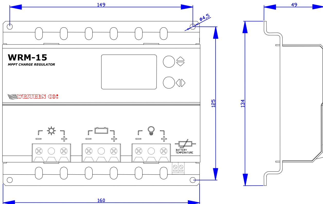
Fig. 8 Dimensioni
