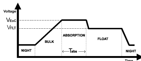
2 Grafico fasi di ricarica:
