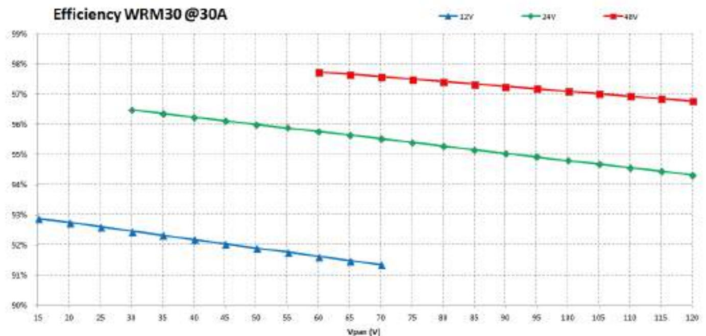
Graf. 2 Efficienze
