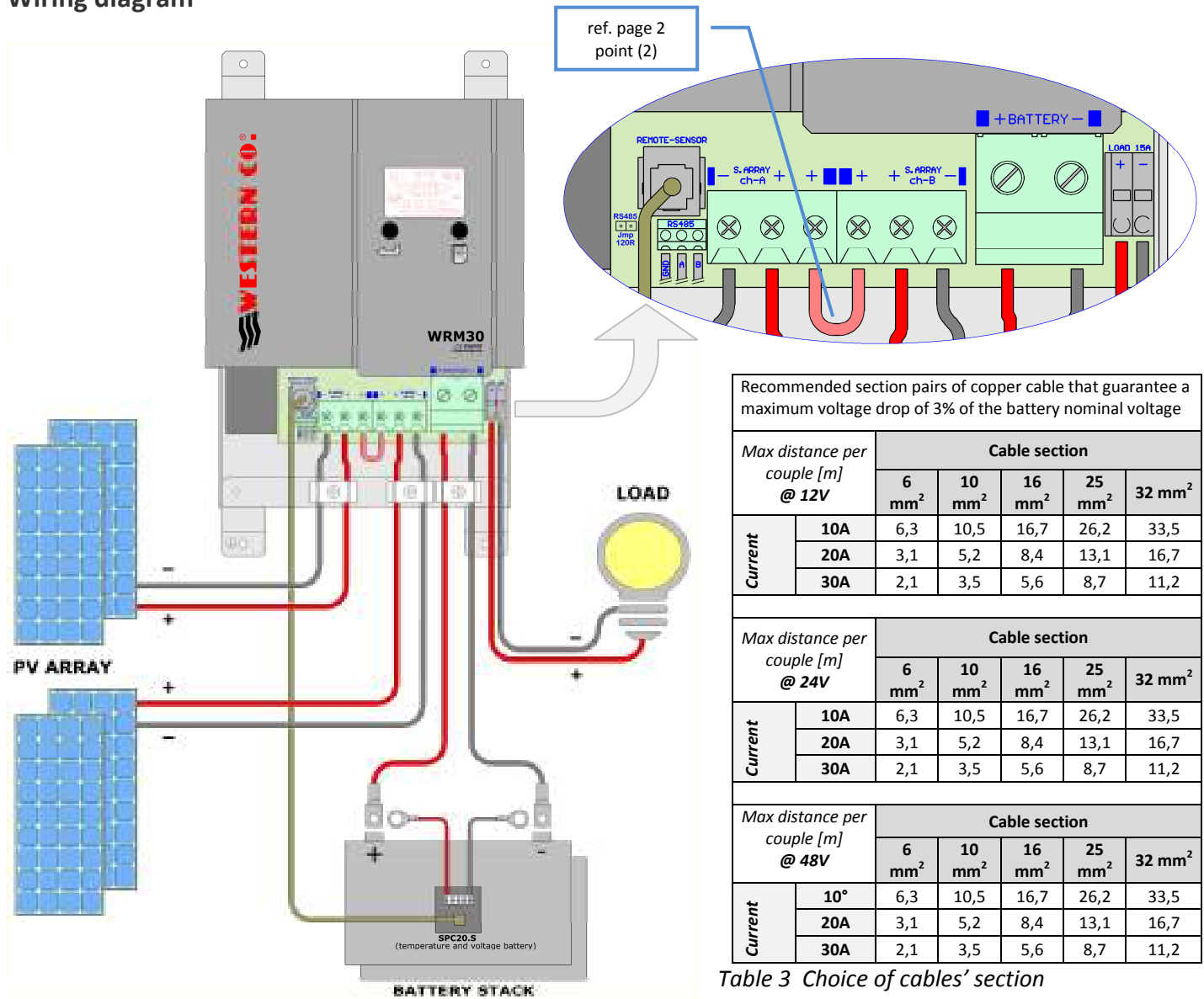
Fig. 2 Wiring diagram
